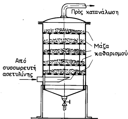
Σχ. 4.2ιγ. Συσκευή καθαρισμού (φίλτρο) ασετυλίνης.
