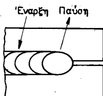
Σχ. 5.8ζ. Θέσεις έναρξεως και παύσεως του τόξου.
