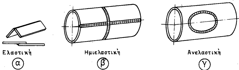
Σχ. 5.6ia. Είδη συνδέσεως.
