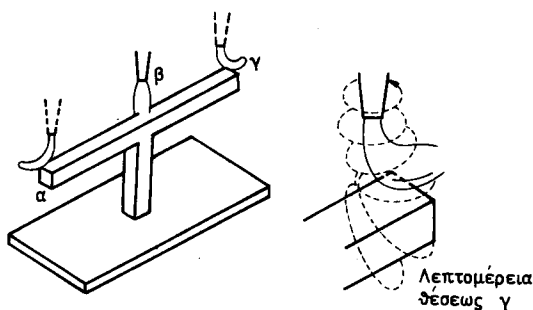
Σχ. 5.26. Μαγνητικό φύσημα του τόξου.
