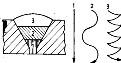
Σχ. 5.8η. Ορθή οδήγηση του τόξου σε ηλεκτρο- συγκόλληση τριών στρώσεων.
