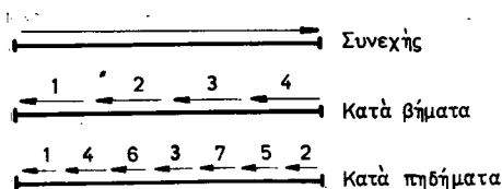
Σχ. 5.6ib. Μέθοδοι ηλεκτροσυγκολλήσεως.
