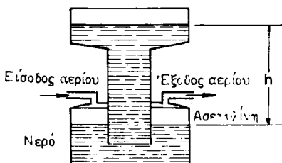
Σχ. 4.2ια. Συσσωρευτής ασετυλίνης μέσης πίεσεως.
